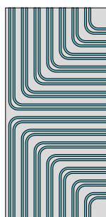
Floortherm Sarokelem 1250x600 mm, a csővezetések ka- nyarodását segíti, panelenként 2x7 sarok alakítható ki belőle
